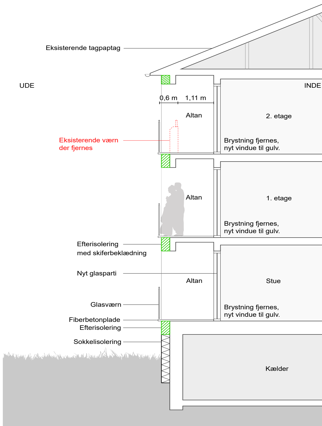
Principsnit, der viser fremtidige forhold - dybere altaner og vindue til gulv
