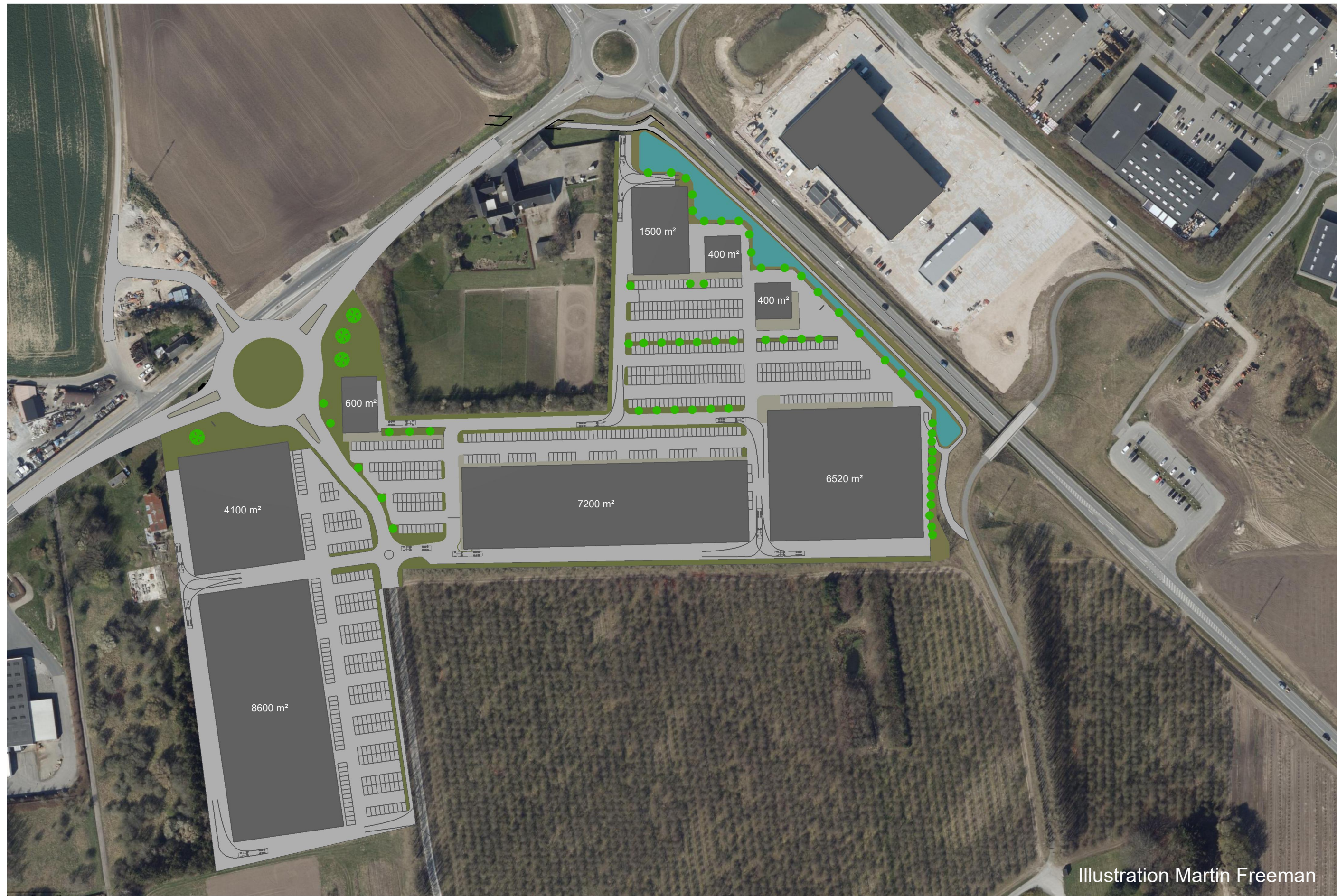
Situationsplan med mulig disponering jf. lokalplanens rammer
