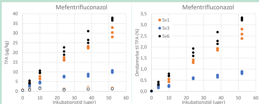
FIGUR 10. Omdannelse af mefentrifluconazol til TFA i tre økologiske landbrugsjorde (Sv1, Sv3 og Sv6). Til venstre er dannelsen vist i absolutte koncentrationer ( n=3 ) med angivelse af koncentrationer i ikke-spikede kontroller (åbne symboler, n=1 ). Til højre er koncentrationer fratrasket baggrunds niveauer og vist i procent af moderstoffets potentielle TFA-ækvivalenter.
