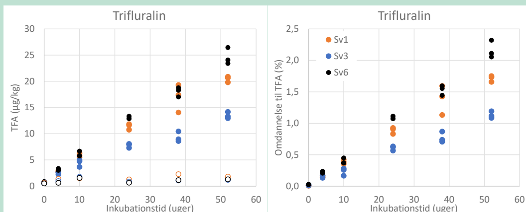
FIGUR 11. Omdannelse af trifluralin til TFA i tre økologiske landbrugsjorde (Sv1, Sv3 og Sv6). Til venstre er dannelsen vist i absolutte koncentrationer ( n=3 ) med angivelse af koncentrationer i ikke-spikede kontroller (åbne symboler, n=1 ). Til højre er koncentrationer fratrasket baggrunds niveauer og vist i procent af moderstoffets potentielle TFA-ækvivalenter.
