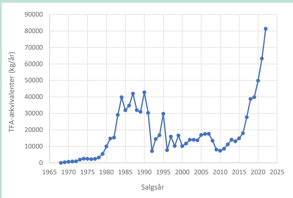
FIGUR 5. Solgte C-CF 3 pesticidmængder omregnet til potentielle TFA-ækvivalenter.
