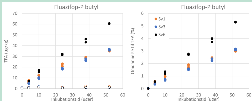
FIGUR 9. Omdannelse af fluazifop-p-butyl til TFA i tre økologiske landbrugsjorde (Sv1, Sv3 og Sv6). Til venstre er dannelsen vist i absolutte koncentrationer ( n=3 ) med angivelse af koncentrationer i ikke-spikede kontroller (åbne symboler, n=1 ). Til højre er koncentrationer fratrasket baggrunds niveauer og vist i procent af moderstoffets potentielle TFA-ækvivalenter.
