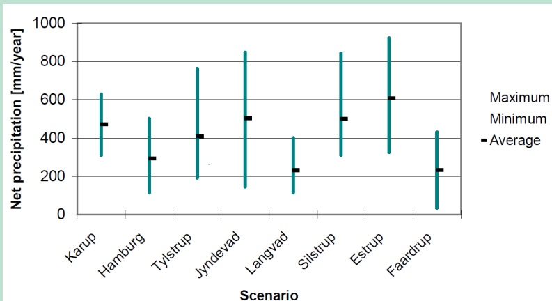
FIGUR 13. Nettonedbør for marker beliggende forskellige steder i Danmark sammenlignet med Hamborg-scenariet. Nettonedbøren er angivet som årlig middelværdi, maksimum og minimum i en 20-års periode. Karup og Langvad har tidligere indgået i Miljøstyrelsens modelberegninger. Tylstrup, Jyndevad, Silstrup, Estrup og Faardrup er marker i Varslingssystem for Udvaskning af Pesticider til Grundvandet (VAP). Figuren er oprindeligt vist i Barlebo et. al. (2007).
