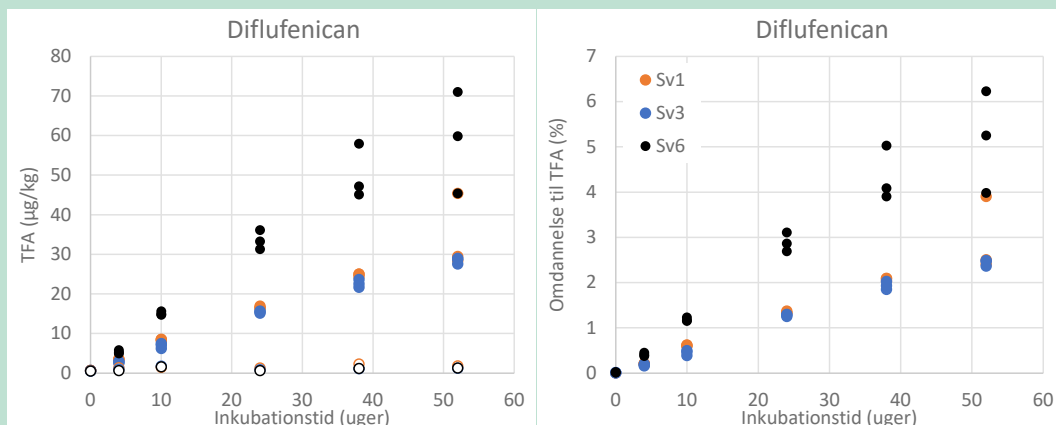
FIGUR 8. Omdannelse af diflufenican til TFA i tre økologiske landbrugsjorde (Sv1, Sv3 og Sv6). Til venstre er dannelsen vist i absolutte koncentrationer ( n=3 ) med angivelse af koncentrationer i ikke-spikede kontroller (åbne symboler, n=1 ). Til højre er koncentrationer fratrasket baggrunds niveauer og vist i procent af moderstoffets potentielle TFA-ækvivalenter.
