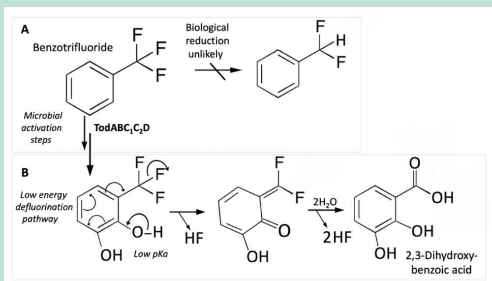
FIGUR 3. Mikrobiel defluorering af benzotrifluorid efter reaktion med toluen-dioxygenase, der introducerer hydroxy-grupper i ortho- og meta-position (Wackett, 2022)
