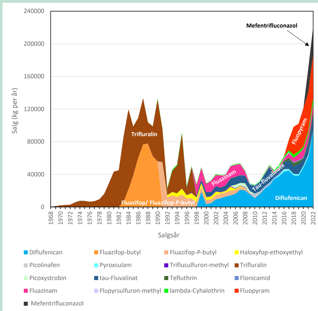
FIGUR 4. Årligt summeret salg af C-CF 3 pesticider ifølge Miljøstyrelsens årlige bekæmpelsesmiddelstatistikker. Figuren viser kun stoffer med et samlet salg i hele salgsperioden >1000 kg
