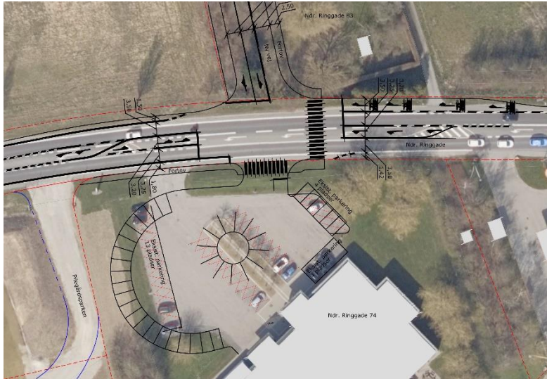
Illustrationen viser et eksempel på et lyskryds samt diverse tilpasninger som fortov, fodgængerfelt mv.
