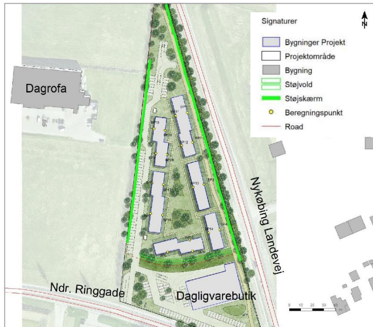
Kortet viser de steder, hvor det er nødvendigt at opstille støjforanstaltninger ved delområde B for at overholde Miljøstyrelsens vejledende grænseværdier.
