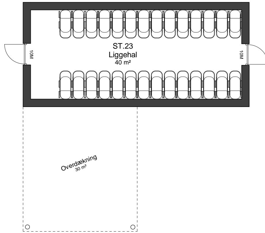
Liggehal 1 : 100
