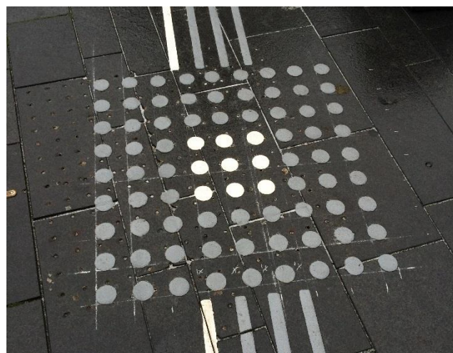
Foto 11: Opmærksomhedsfelt i termoplast, forsøg fra Schweizerpladsen i Slagelse.
