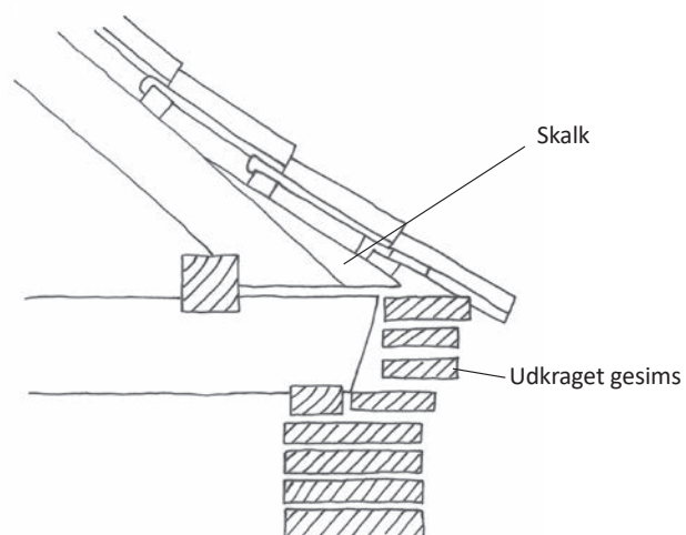
Principiell illustration (snittegning) af en tagkonstruktion med opskalkning og udkraget, muret gesims. Efterisolering på ydersiden af spærene, hvor tagfladen løftes vil forandre tagprofilen markant.
