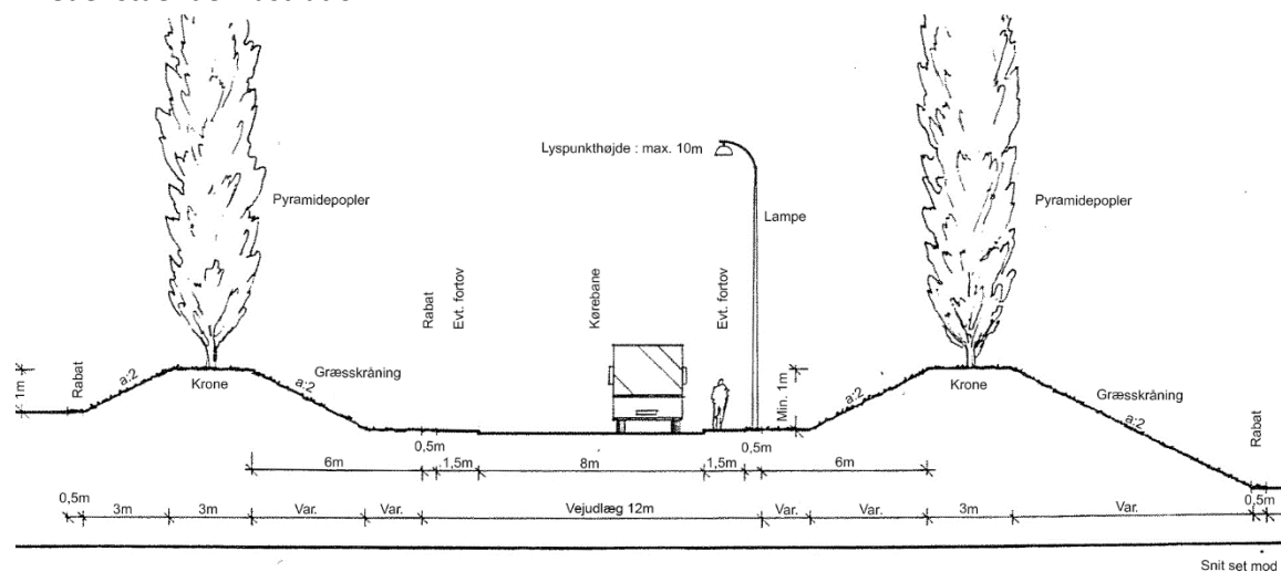
Tværsnit af Trafikcenter Allé gengivet fra Lokalplan 197 og 257, der viser vejprofilen med jordvolde og pyramidepopler på begge sider.
