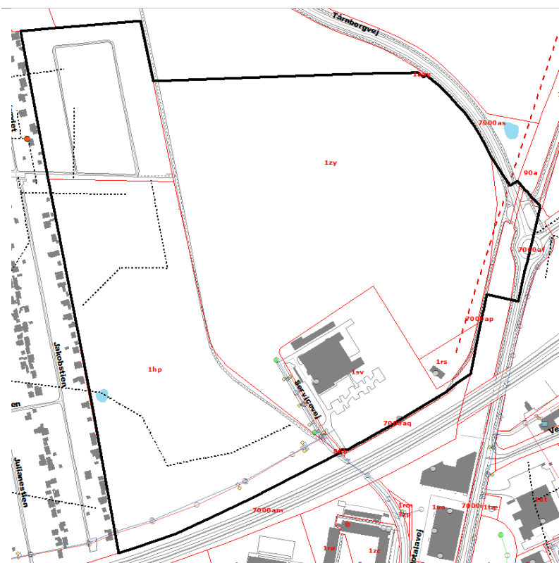
Drænledninger (sort stiplede linje). 50 kv luftledning (rød stiplede linje). Mod syd spildevandsledning og regnvandsledning parrallelt med Vestmotorvejen.
