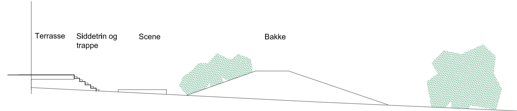
Snit gennem terrasse, siddetrin, scene og kælkebakke ved 'finger 3' mål 1:200
