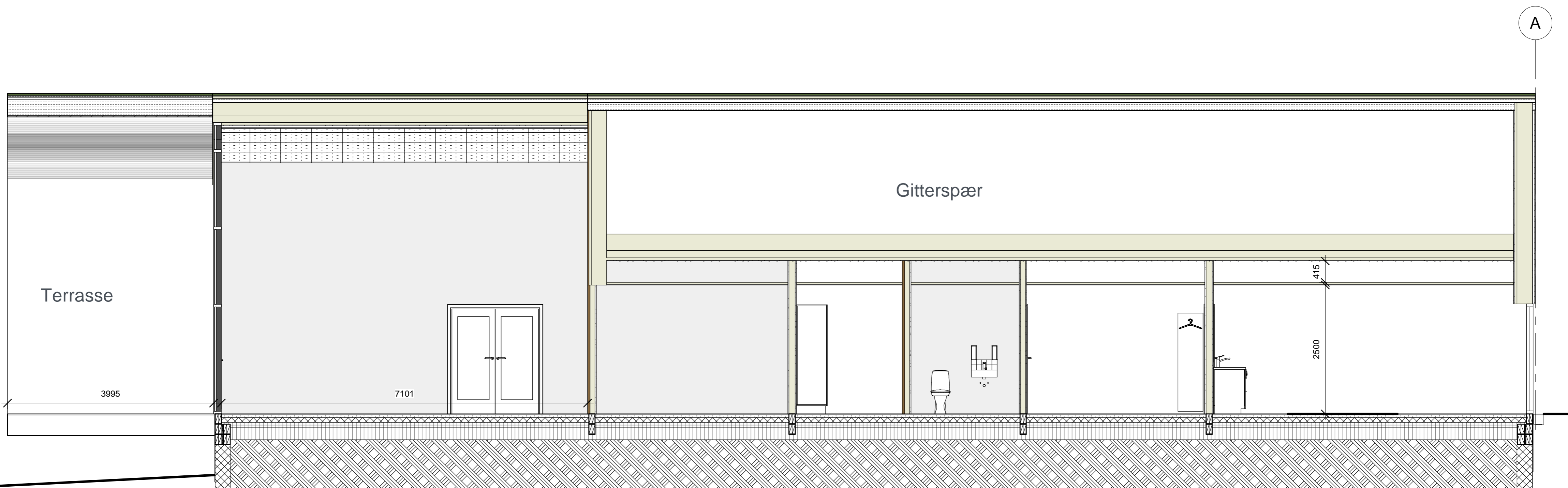
8 Snit 2-2 1 : 50
