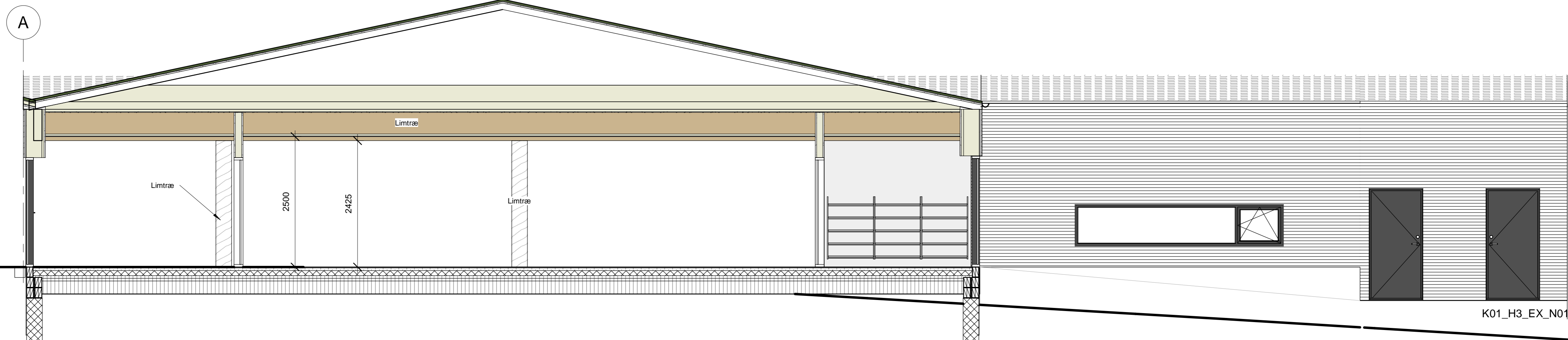
8 Snit 2-2 1 : 50
