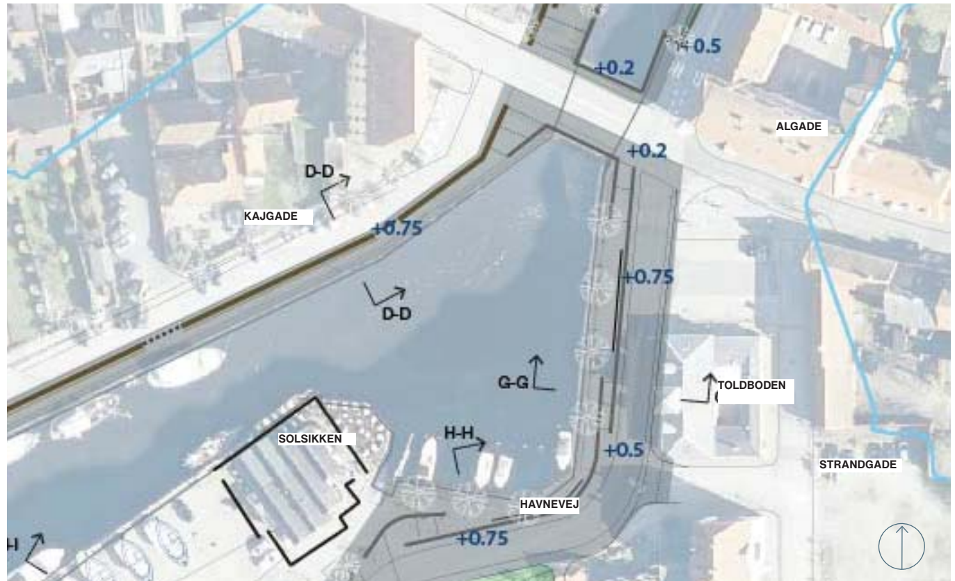
Planudsnit 1:1000
