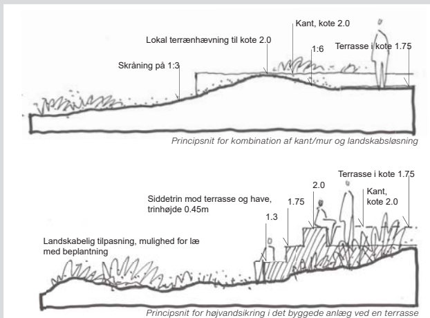
Principsnit for højvandssikring integreret i det haveanlæg. Schönherr
