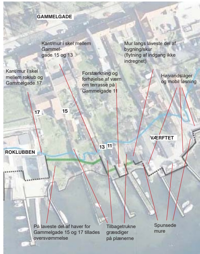
Planudsnit ca. 1:1600
