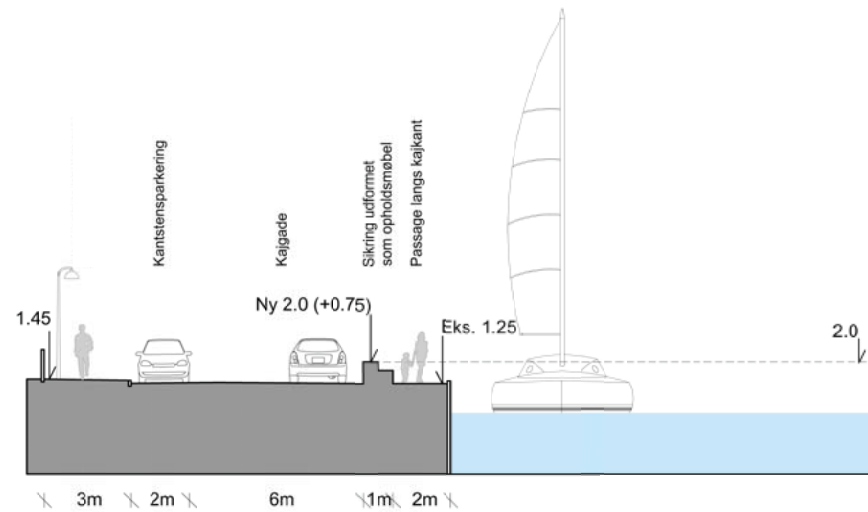
SNIT D-D
