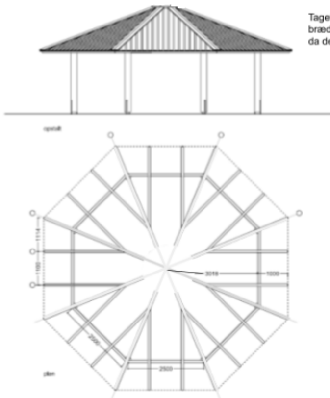
Billede 2. Spærplan og opstalt
