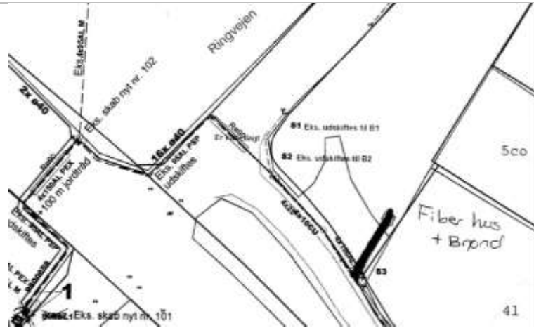
Placering signalkabler til bredbåndsforbindelse. Kabler føres fra Sørby Hovedgade frem til teknikbygning (fiberhus) og underjordisk bredbåndsbrønd på matr. nr. 5cp Sørbymagle by, Sørbymagle.
