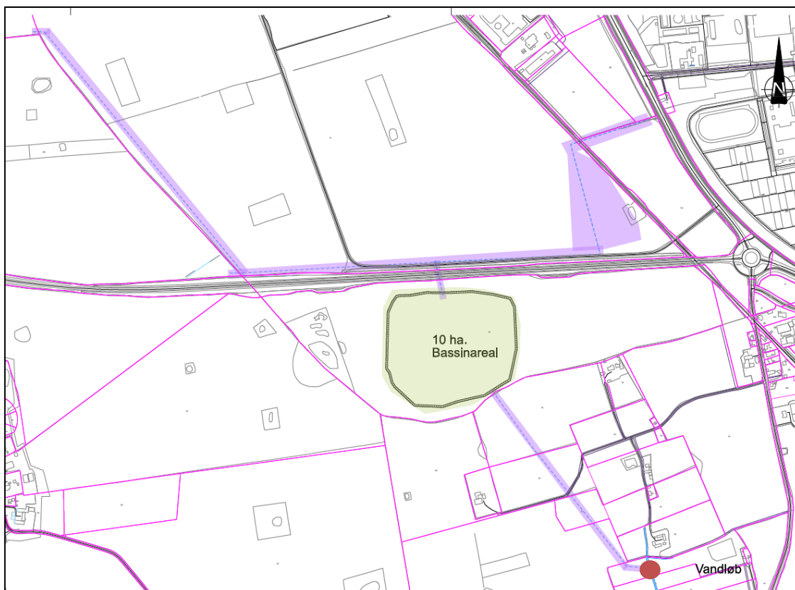
Figur 2: Oversigt over bassinets placering (grøn). Udledningpunktet, på Harrested Å har en rød cirkel. Ledningstraceerne og adgangsveje er angivet med lilla.
