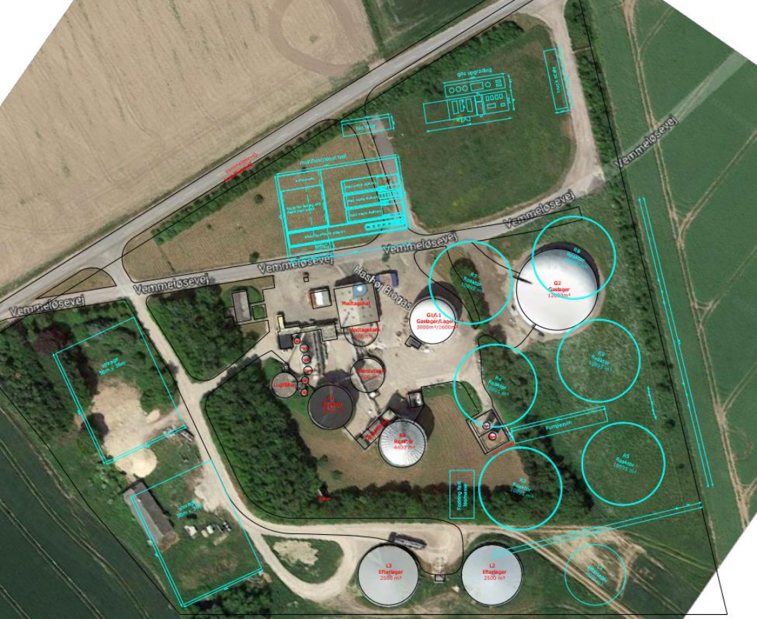
Figur 1.3.2: Skitsetegning for placering af eksisterende og nye anlæg. De planlagte nye anlæg er indtegnet med grøn.
