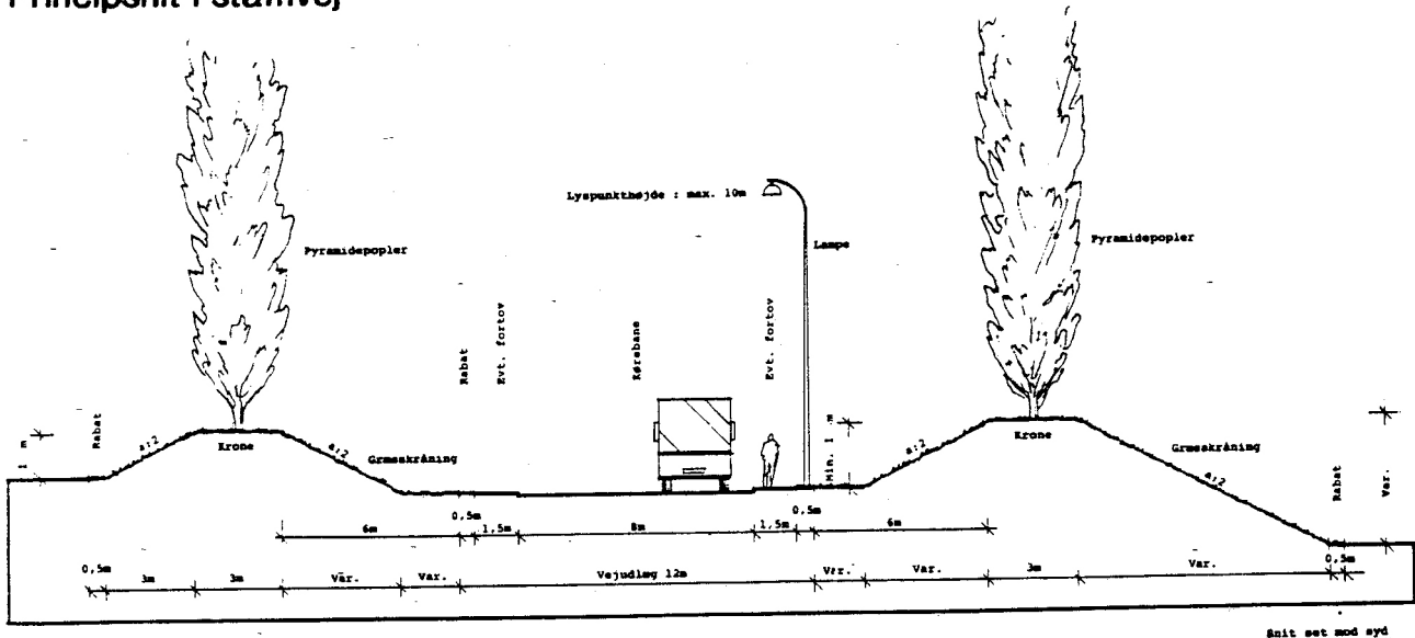
Principsnit i stamvej
