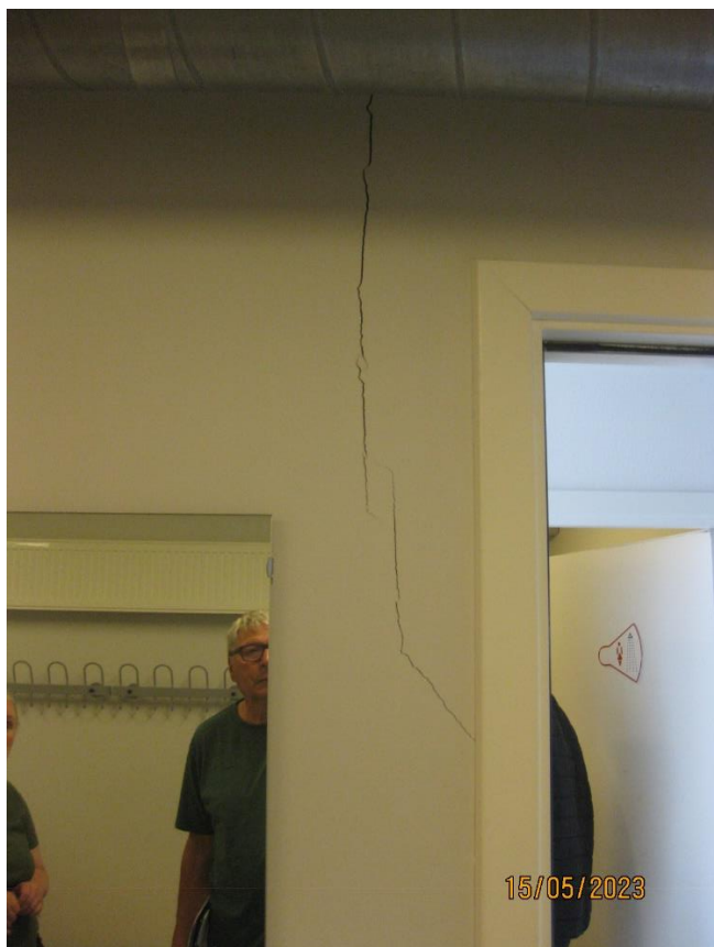
Der forekommer sætningsrevner i skillevægge til omklædningsrummene
