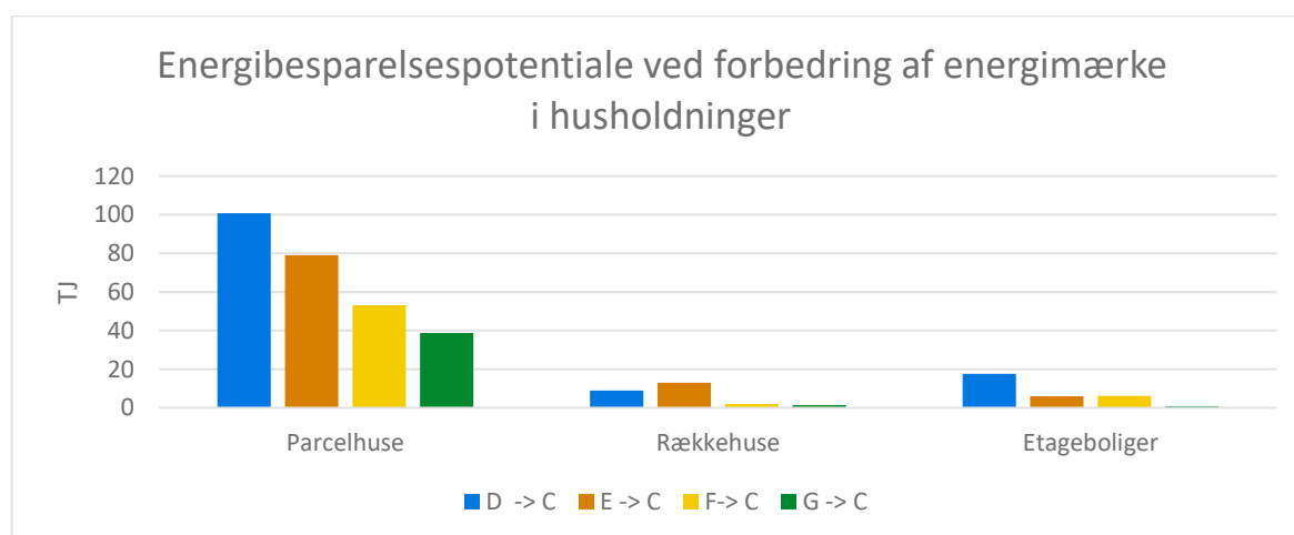
Figur 1 Energibesparelspotentialt ved forbedring af energimærker i husholdninger
