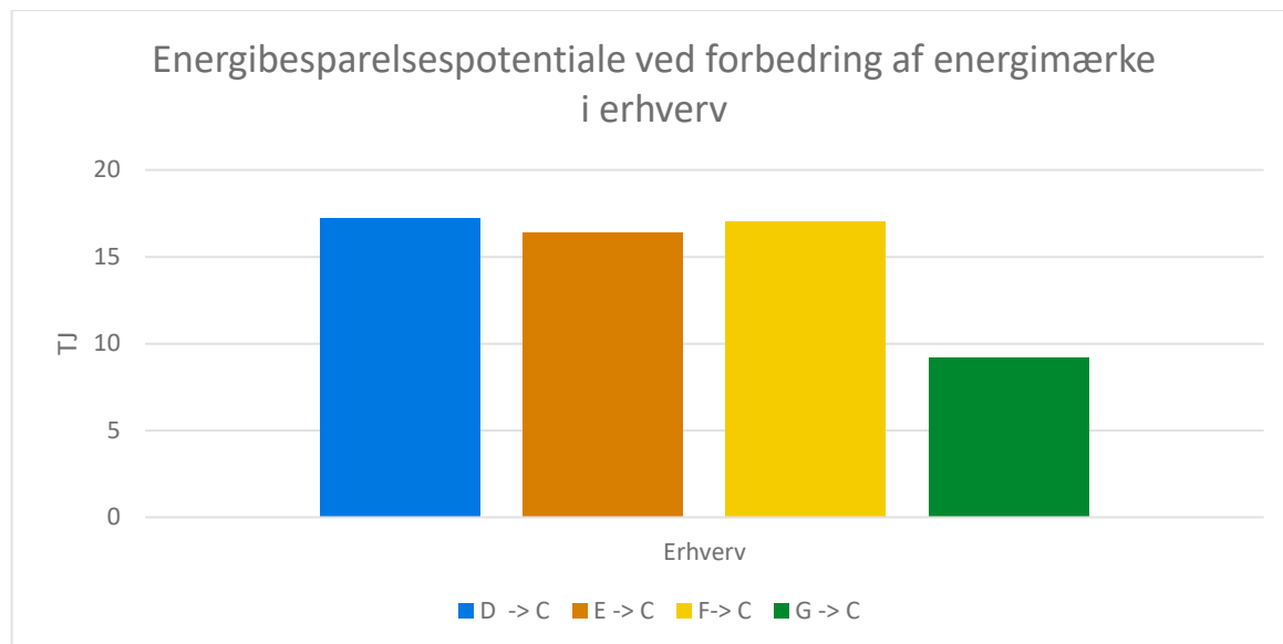
Figur 2 Energibesparelspotentialet ved forbedring af energimærker i erhverv
