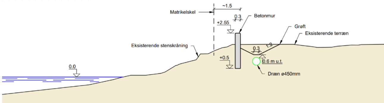
SNIT A-A, 1:100
